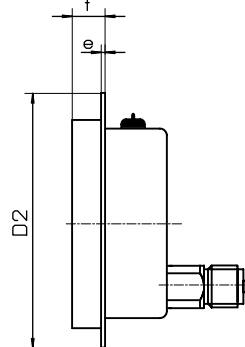
Rand vorn
